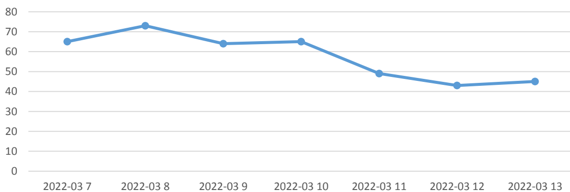
U200sr-średnia dobowa wilgotność powietrza
