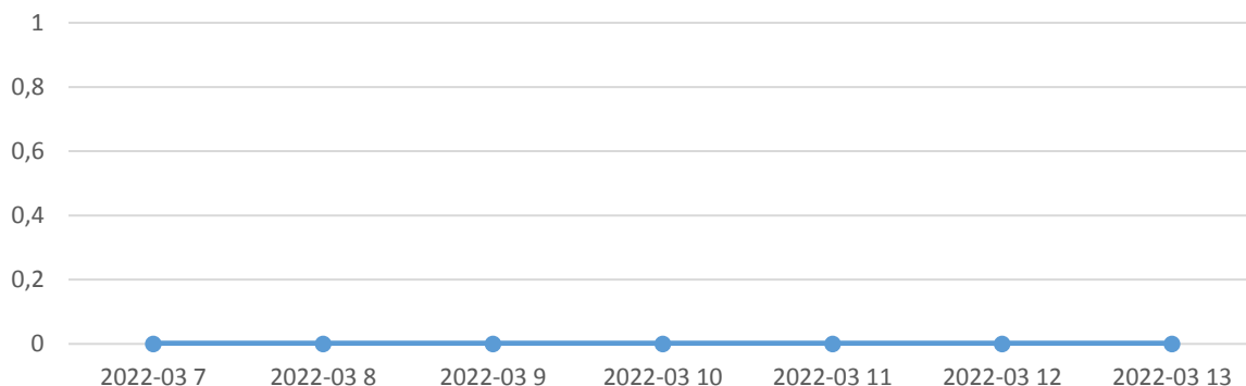
OP1-dobowe opady wody w mm/m kwadratowy
