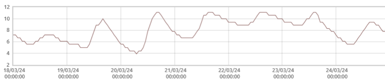
■ Matuszyn: Temperatura gleby [C]
