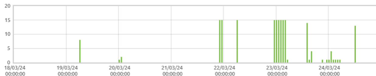
■ Matuszyn: Zwilżenie liścia
