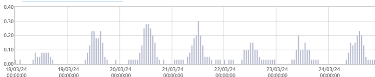
■ Matuszyn: Ewapotranspiracja [mm]
